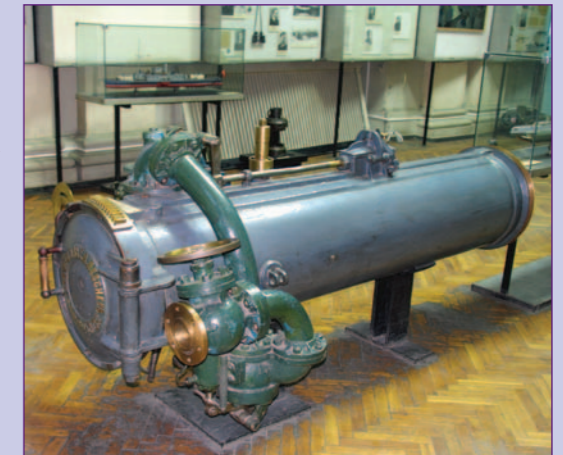
▲ Казенная часть торпедного аппарата подводной лодки «Пантера». В августе 1919 года торпедой, выпущенной из этого аппарата, был потоплен в Финском заливе эсминiec «Виттория» британских интервентов
